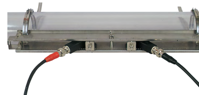
Capteur (FSSA)
