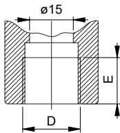
DÉTAIL "B"
