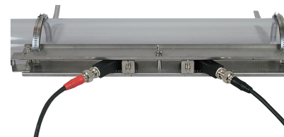
Capteur (FSSA)
