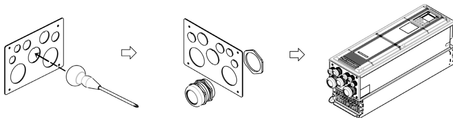
Figure 2.4 Poinçonnement des sections semi-perforées dans la plaque de câblage et montage des presse-étoupes ou des conduites
