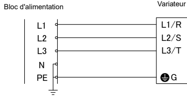
Système TN-S
