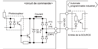
(b) PLC servant comme SOURCE
