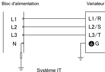
Système IT
