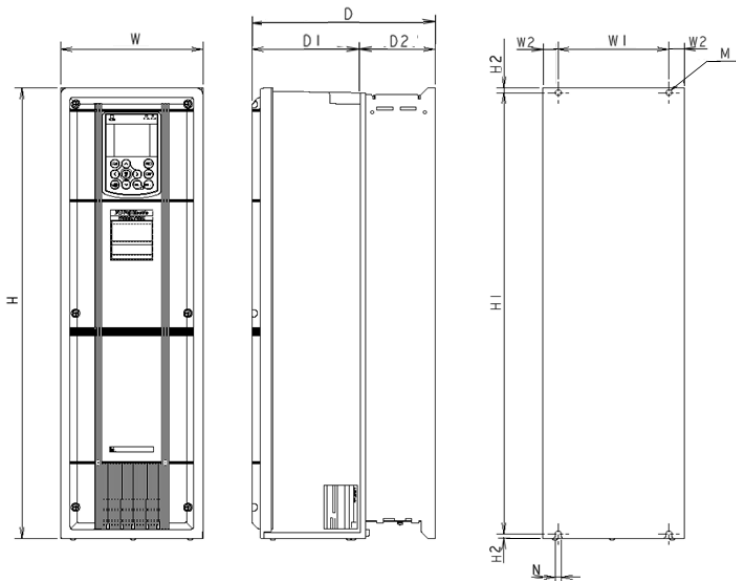
Figure 1 Dimensions extérieures du variateur
