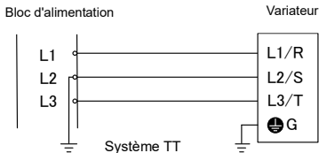
Système TT
