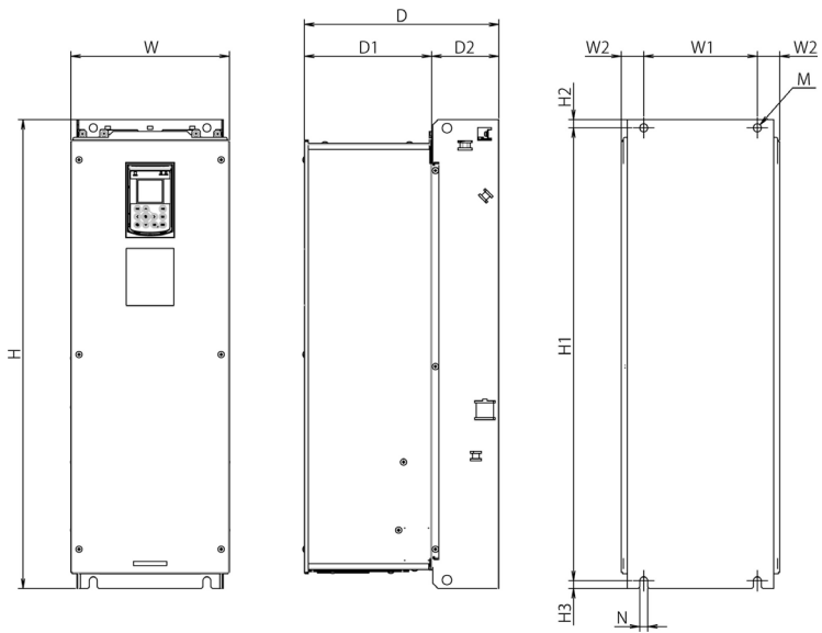
Figure 2 Dimensions extérieures du variateur
