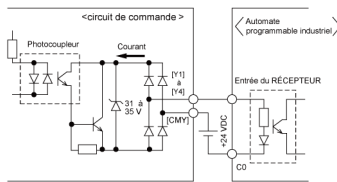
(a) PLC servant comme RÉCEPTEUR
