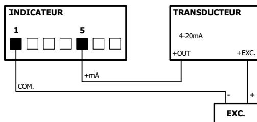
RACCORDEMENT A 2 FILS AVEC EXCITATION EXTERNE
