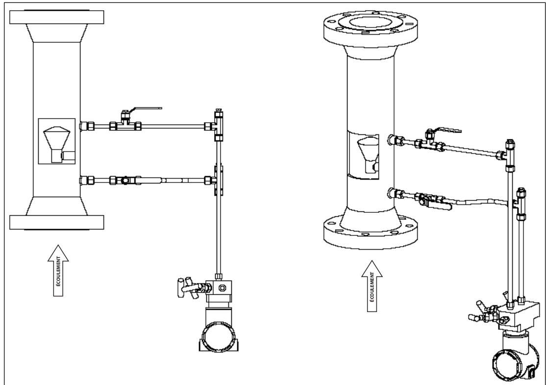
Figure 16. Installation sur Tuyauterie Verticale (Flux Ascendant) pour une Application Impliquant une Vapeur qui se Condense
