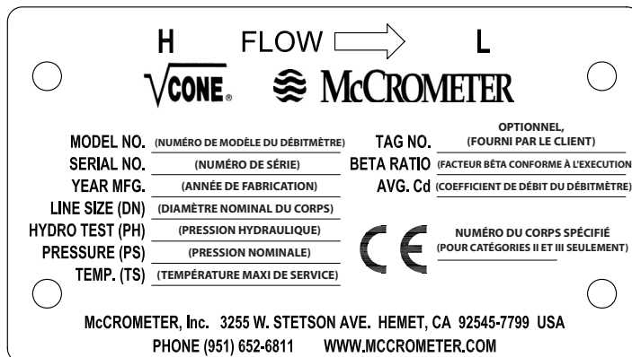
Figure 11. Exemples des Étiquette du Débitmètre
