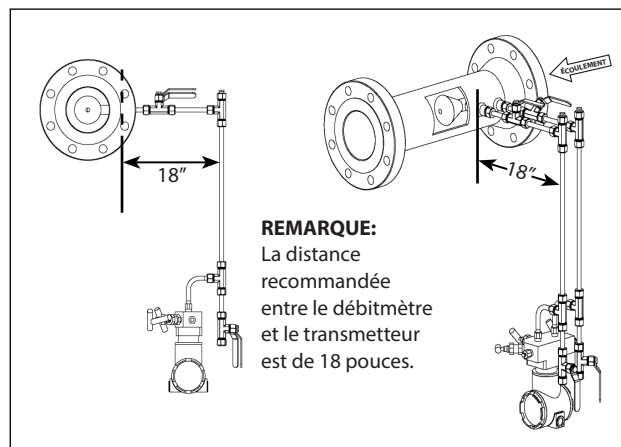
Figure 15. Installation sur Tuyauterie Horizontale pour une Application Impliquant de la Vapeur qui se Condense
