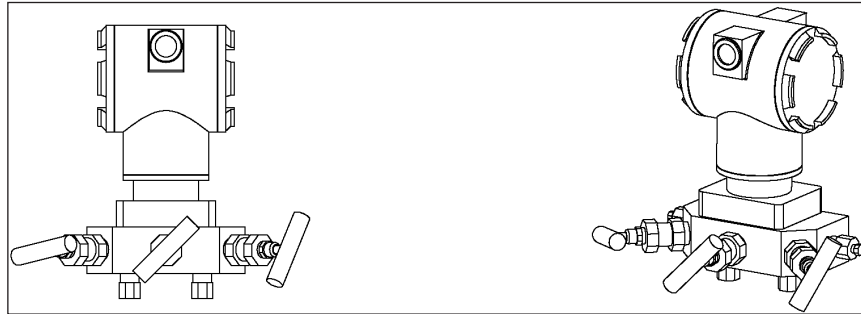
Figure 14. A Un Manifold à Trois Voies Monté avec un Transmetteur de Pression Différentielle
