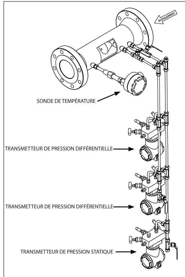
Figure 18. Technique de Montage de Transmetteurs de Pression Différentielle Doubles
