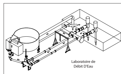
Figure 7. Installation de Calibrage 40k Gravimétrique
