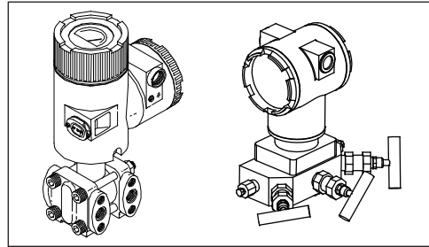
Figure 9. Transmetteur de Pression Différentielle Type avec Manifold de Vannes
