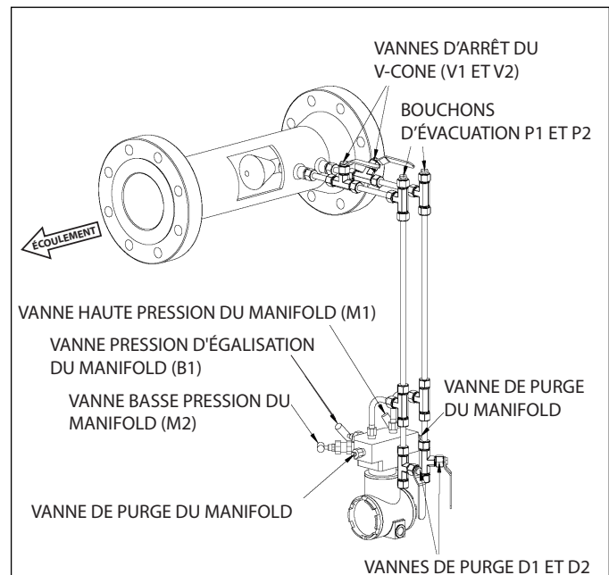
Figure 19. Calibrage du Transmetteur pour Application Impliquant une Vapeur
