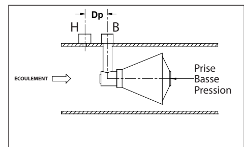
Figure 12. Prises Basse et Haute Pression
